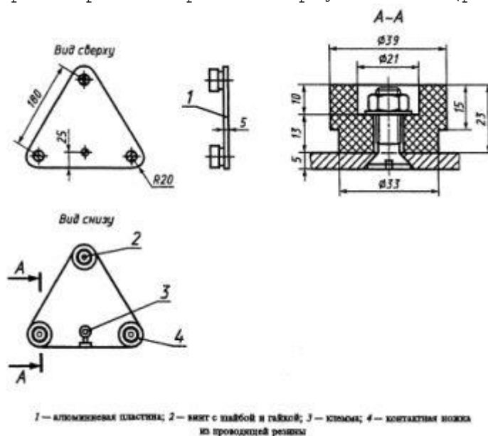
Рисунок А.1 — Испытательный электрод 2
