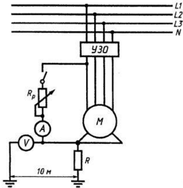
Рисунок В.3 — Схема проверки УЗО по методу 3
