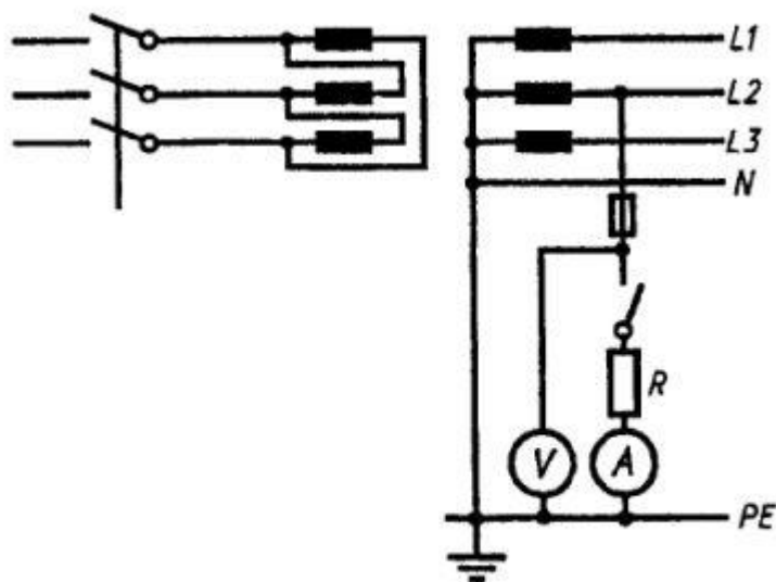
Рисунок D.1 — Схема измерения по методу 1
