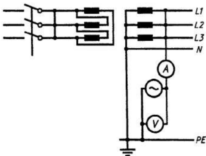
Рисунок D.2 — Схема измерения по методу 2
