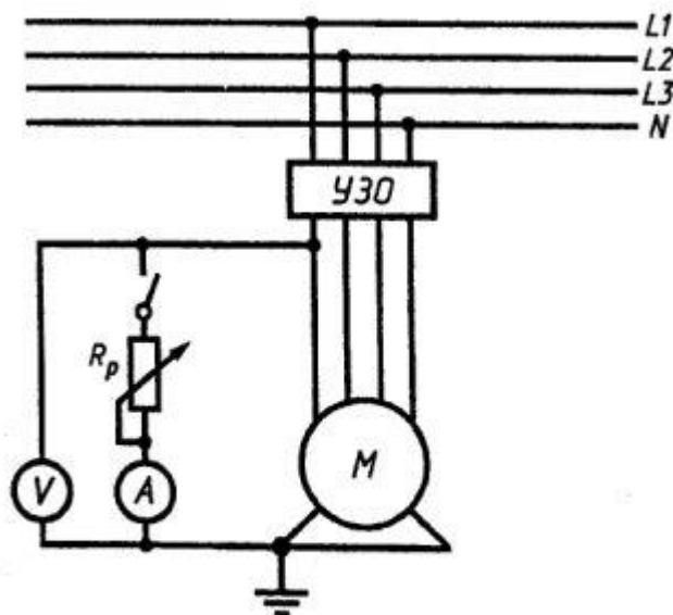
Рисунок В.1 — Схема проверки УЗО по методу 1
