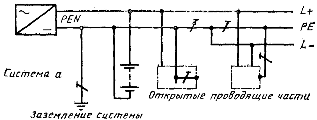
Рисунок 31G - Система TN-C постоянного тока
