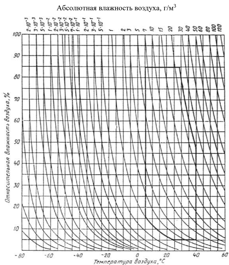
Климатограмма зависимости относительной и абсолютной влажности воздуха от температуры Класс АВ5
