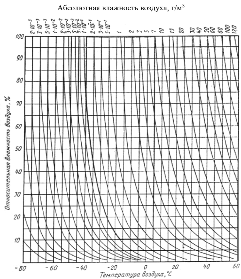
Климатограмма зависимости относительной и абсолютной влажности воздуха от температуры Класс АВ2
