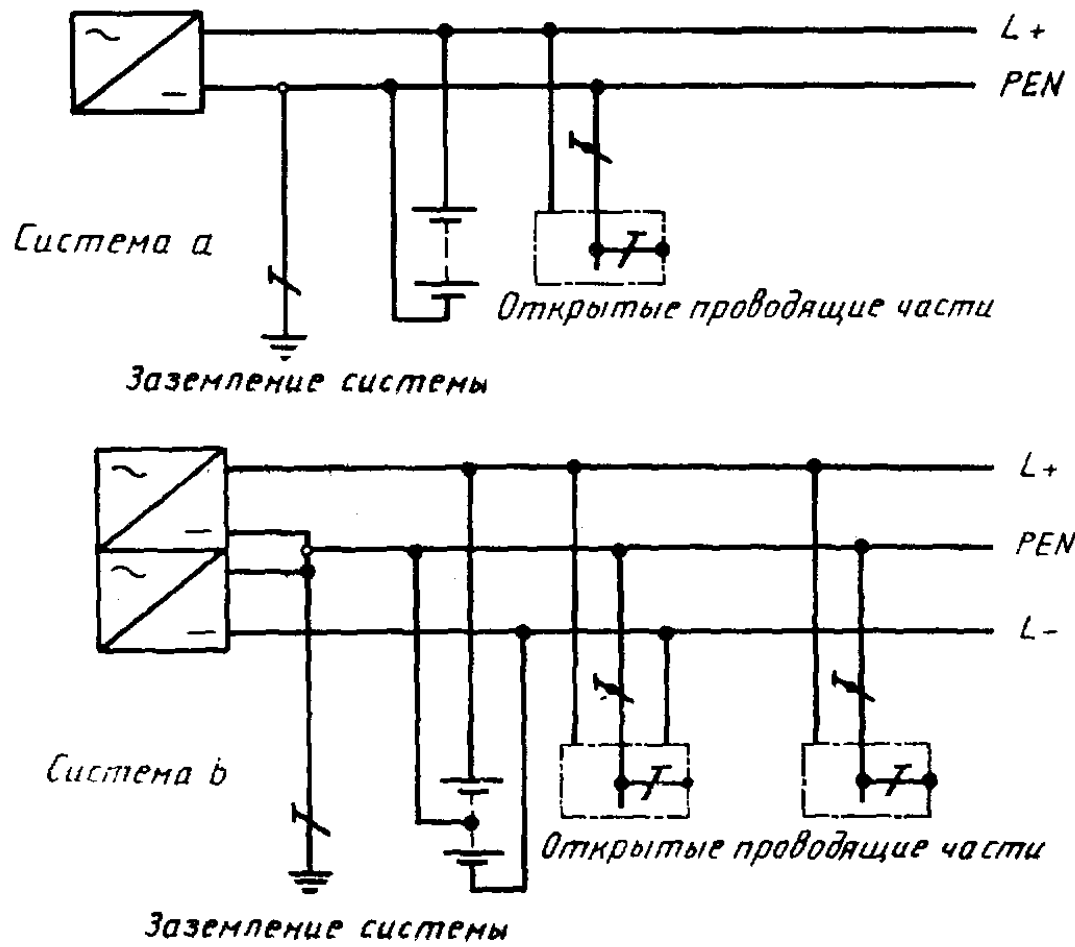
Рисунок 31G - Система TN-C постоянного тока
