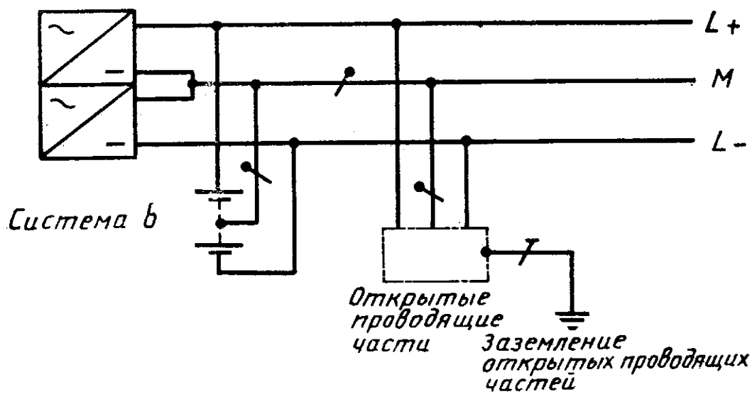
Рисунок 31K - Система IT постоянного тока
