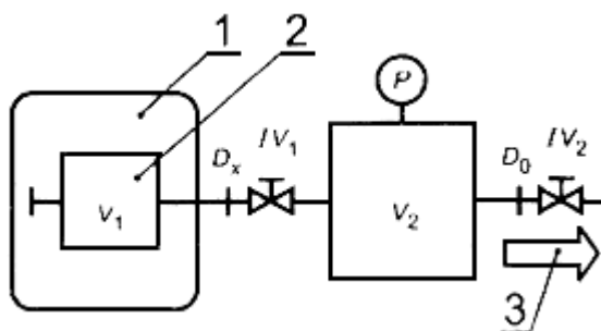
1 - система, заполненная гелием; 2 - испытываемая система; 3 – выход
