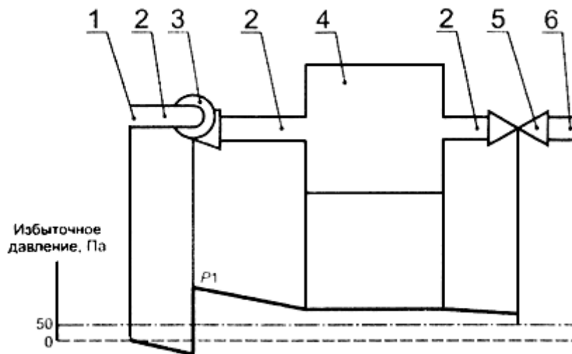
Рисунок В.1б - Выход защитного газа с использованием защитного барьера от искр и частиц
