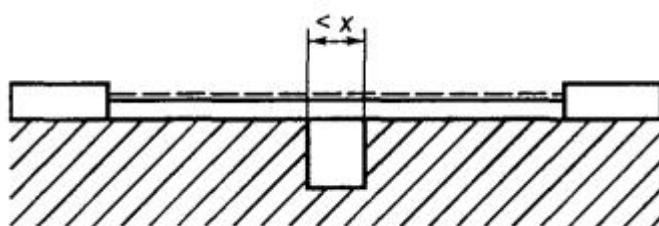
Рисунок Е.1 - Размеры ребер
