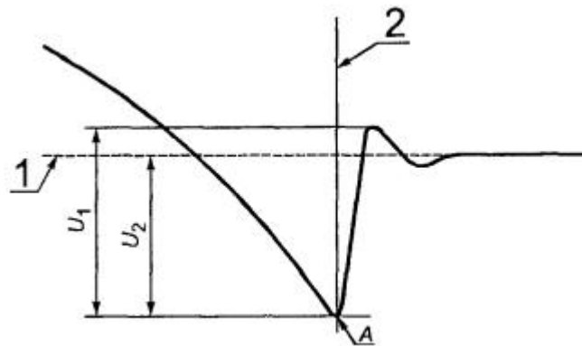
1 - линия развертки; 2 - момент нулевого тока; A - начальная точка
