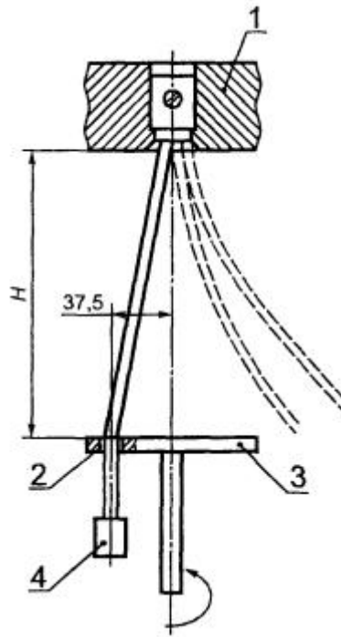
1 - панель; 2 - гильза; 3 - диск; 4 - груз
