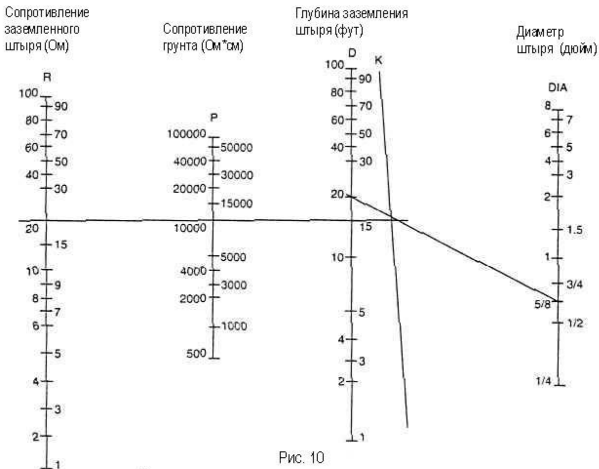
Номограмма для расчета заземления в виде штыря
