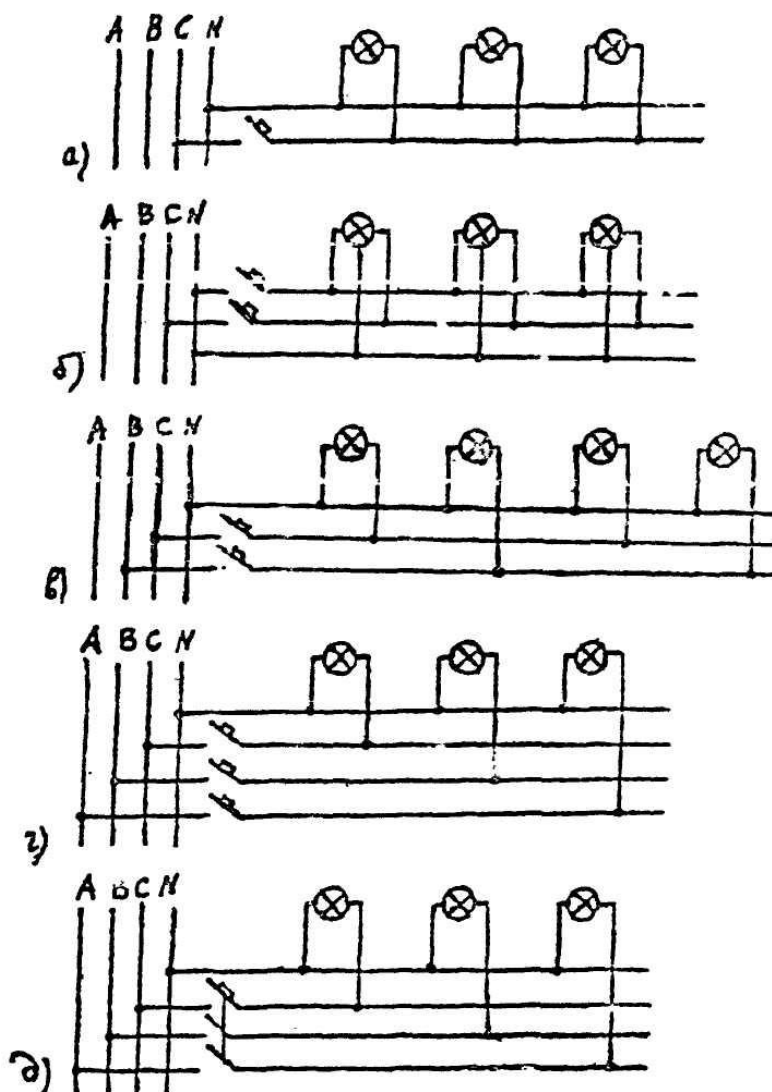
Рис.1. Схемы групповых линий при системах напряжения 660/380, 380/220 и 220/127 В и питания ОП напряжением соответственно 380, 220 и 127 В. а - двухпроводная однофазная; б - трехпроводная однофазная для взрывоопасных зон класса В-I (только для 380/220 и 220/127 В); в - трехпроводная двухфазная; г, д - четырехпроводная трехфазная.
