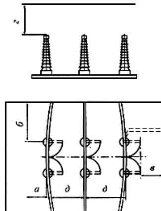
Рис.4.2.1. Границы расположения открытых подвижных контактов разъединителя
