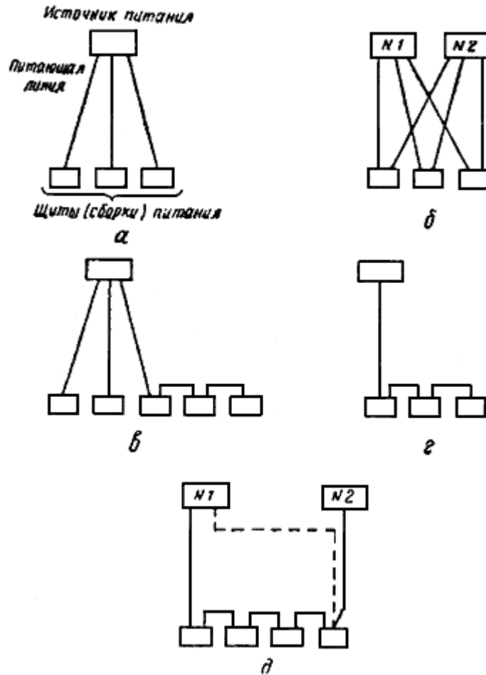
Рис.2. Схема питающей сети системы электропитания:
