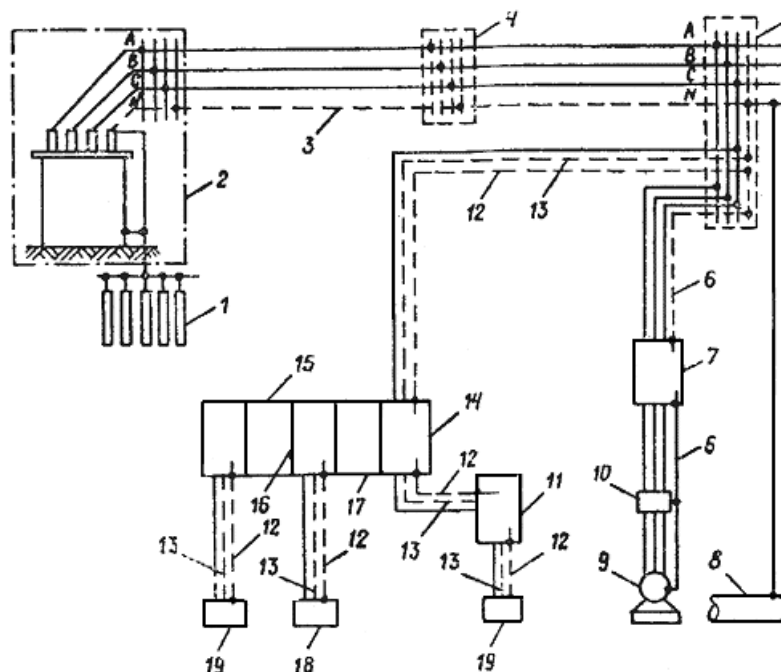
Рис.3. Пример выполнения зануления в электроустановке системы автоматизации:
